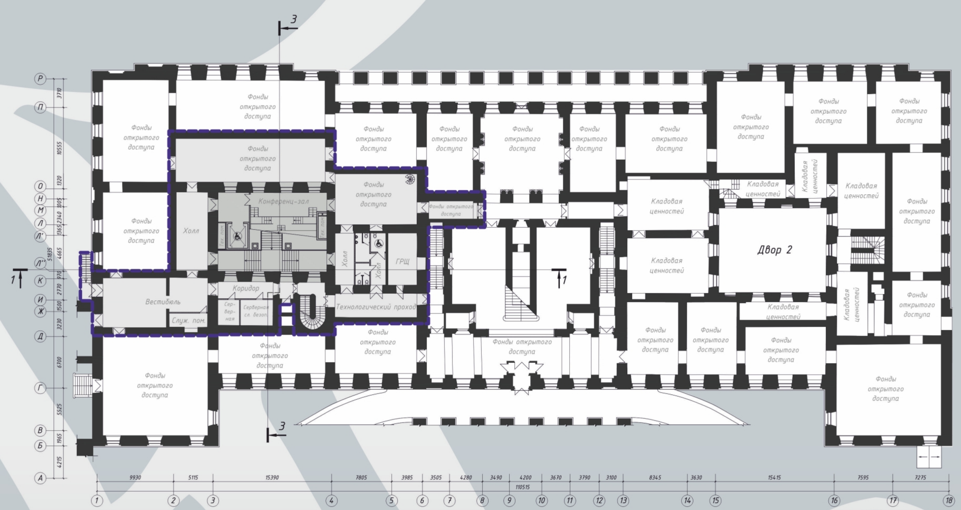
ПЛАН ПЕРВОГО ЭТАЖА
