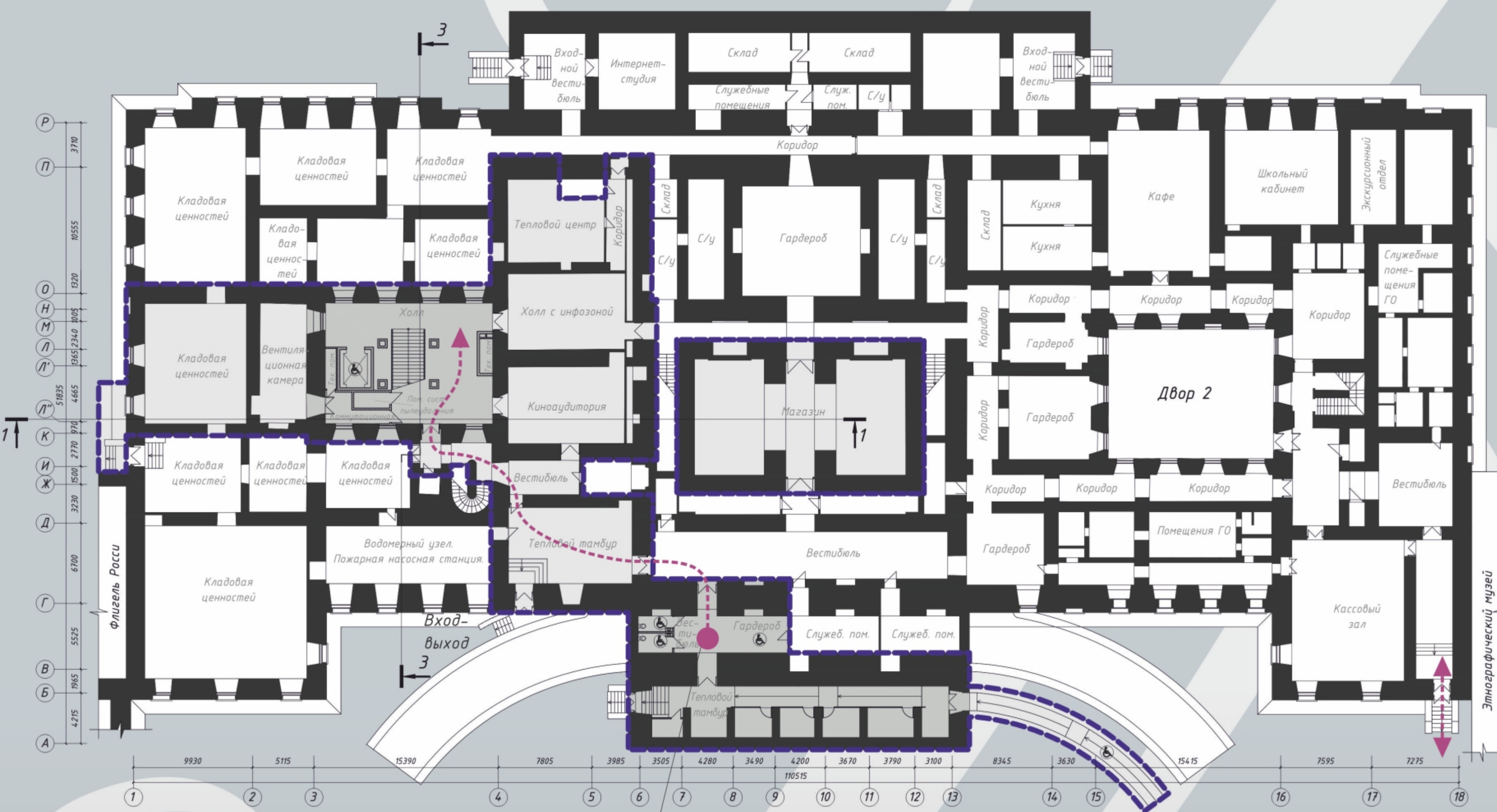
ПЛАН ЦОКОЛЬНОГО ЭТАЖА
